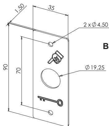
BOPO - P z LED lub bez - avec ou sans LED - with or without LED - mit oder ohne LED
