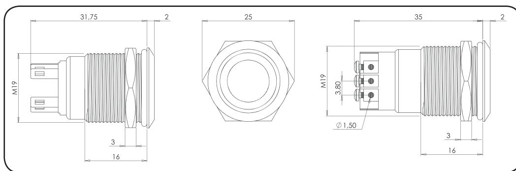
BOPO - P z LED lub bez - avec ou sans LED - with or without LED - mit oder ohne LED
